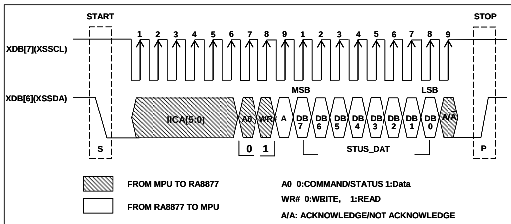
圖 7-23 : Status Read on IIC-Bus
