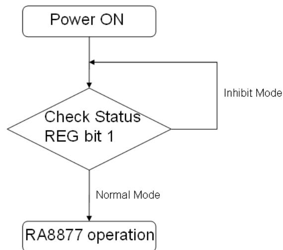
Figure 6-4：開機後，使用 RA8877 必須先檢查 Status REG bit 1 狀態
