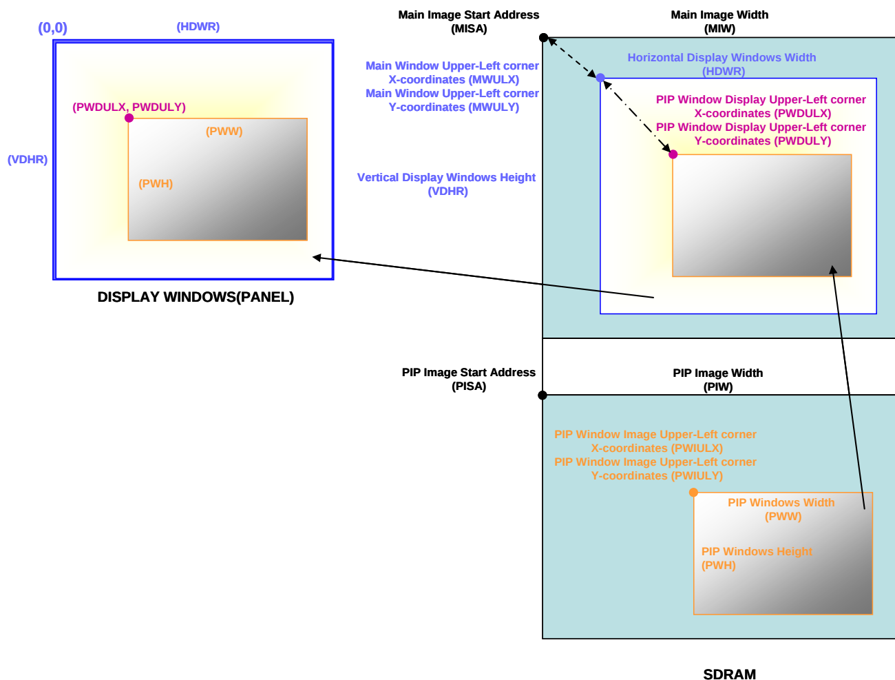
圖 19-2 : LCD Display
