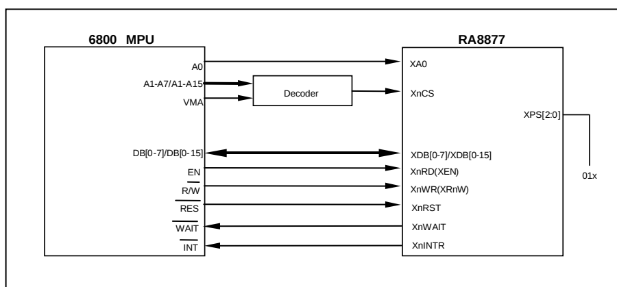
圖 7-2 : 6800 MPU Interface
