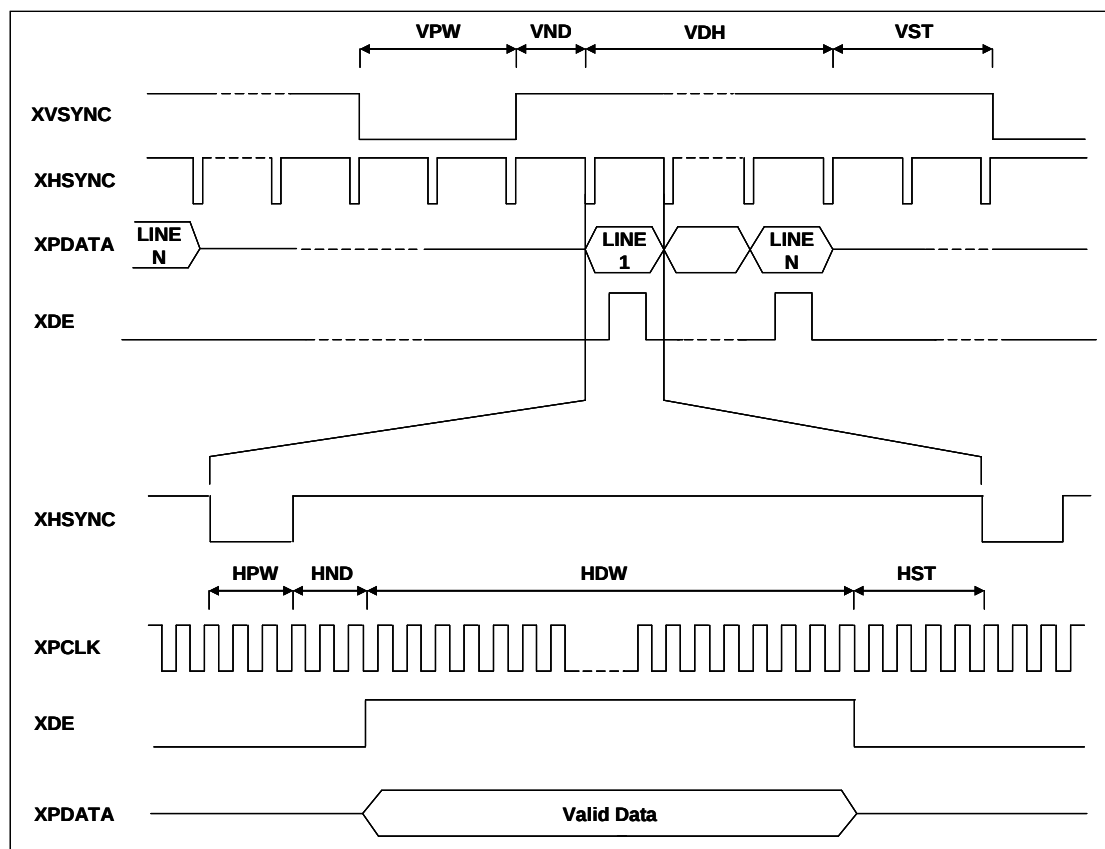
圖 10-1 : Digital TFT Panel Timing
