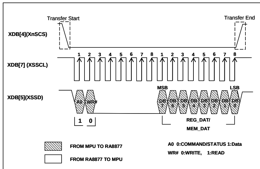
圖 7-11 : Data Write on 3-Wire SPI-Bus
