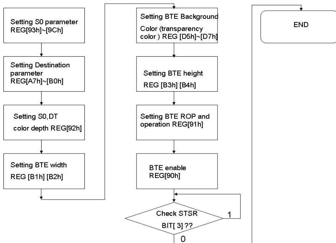
圖 13-12 : Flow Chart
