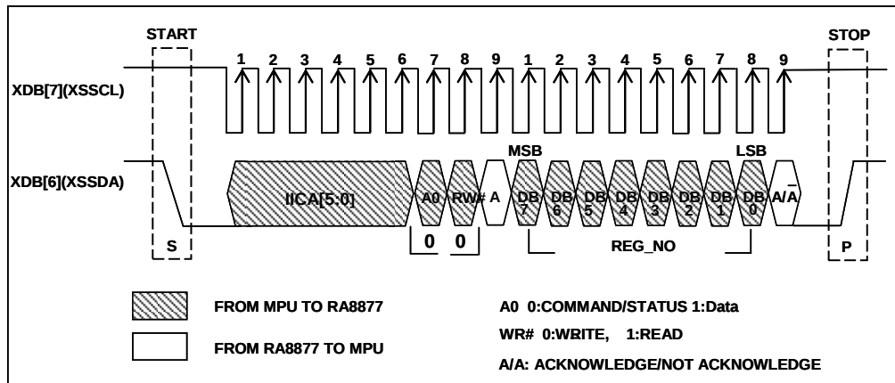
圖 7-22 : CMD Write on IIC-Bus
