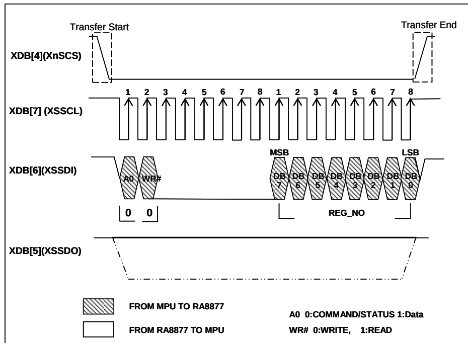
圖 7-16 : CMD Write on 4-Wire SPI-Bus
