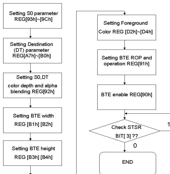
圖 13-38 : Flow Chart
