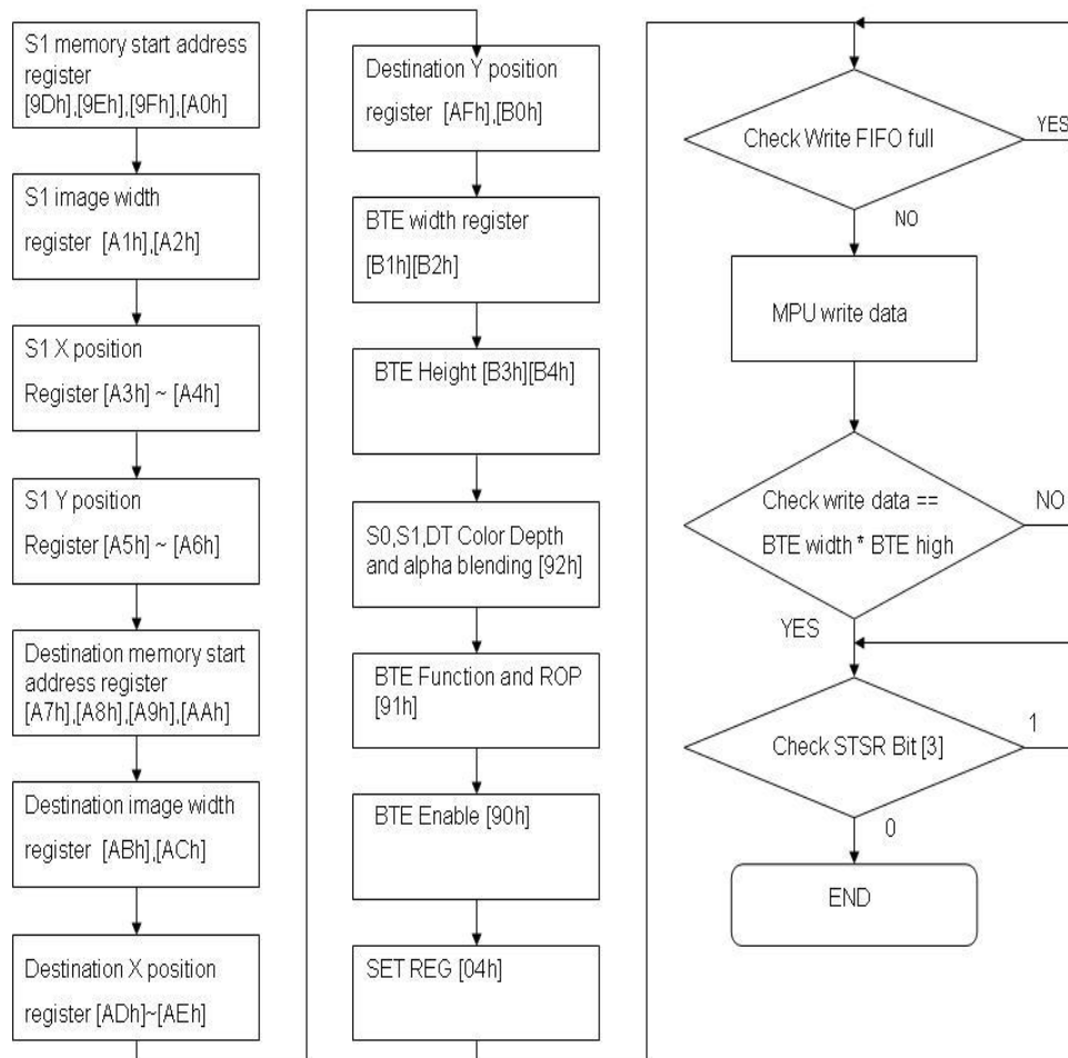
圖 13-6 : Flow Chart
